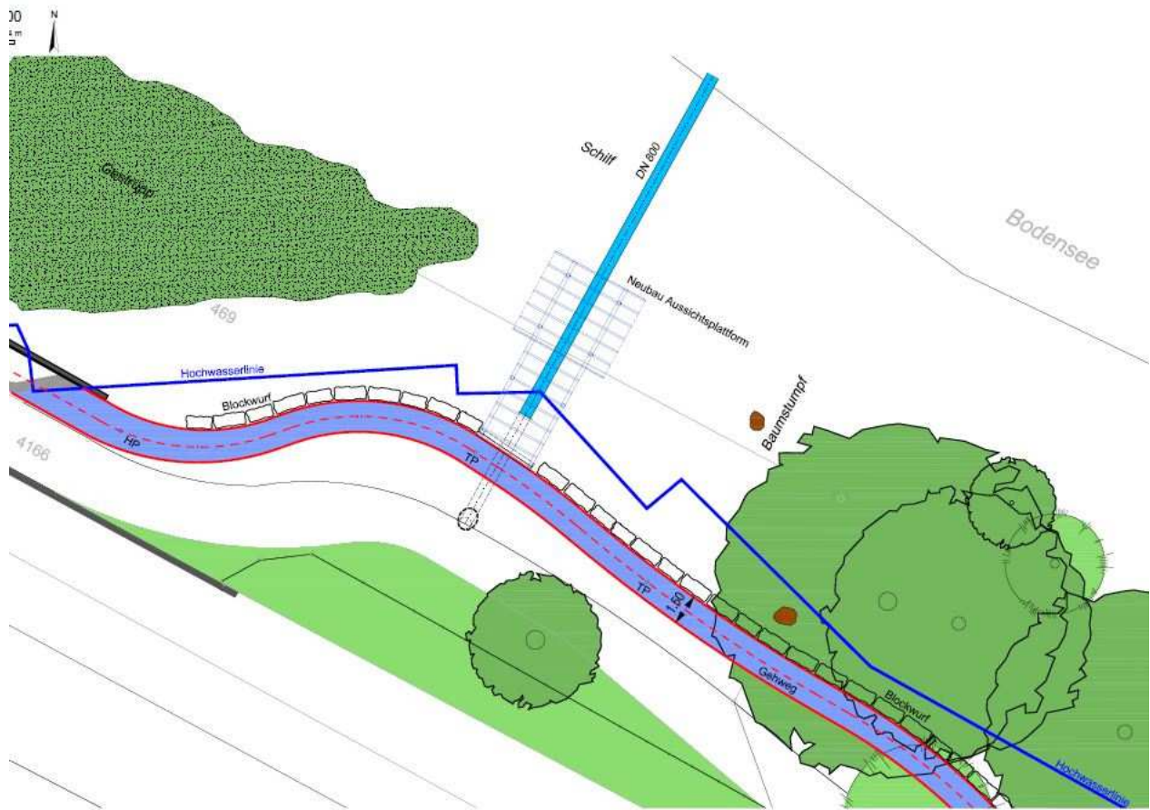
Plan der neuen Fussgängerplattform am Philosophenweg
