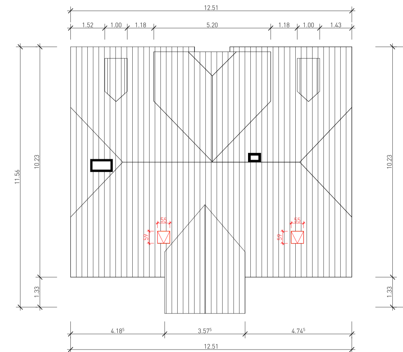
DACHAUFSICHT MST. 1:100
