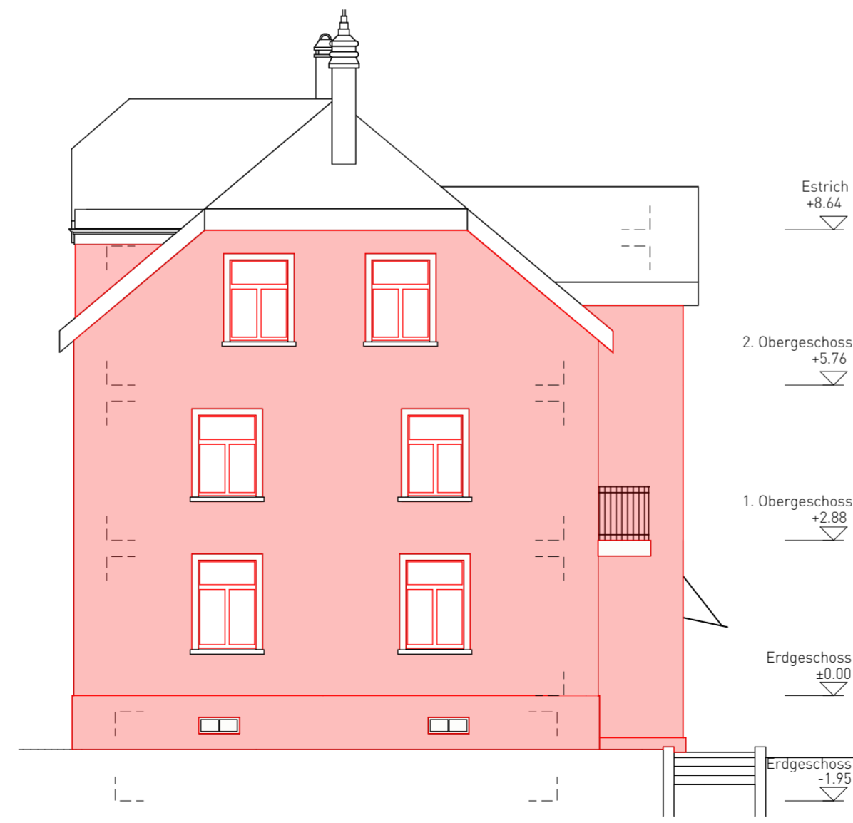
WESTFASSADE MST. 1:100
