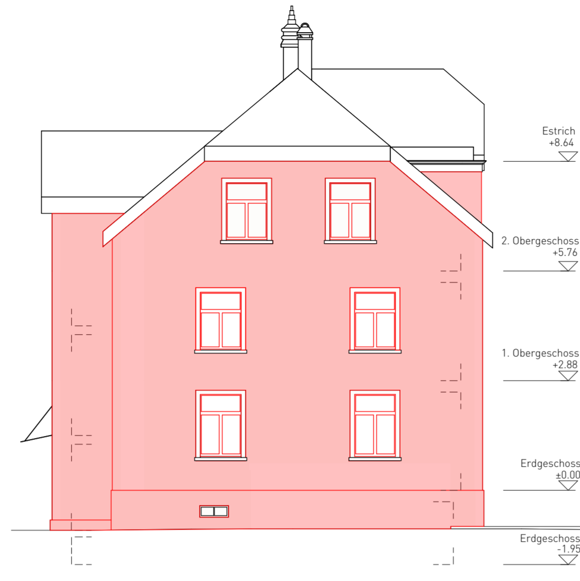
OSTFASSADE MST. 1:100
