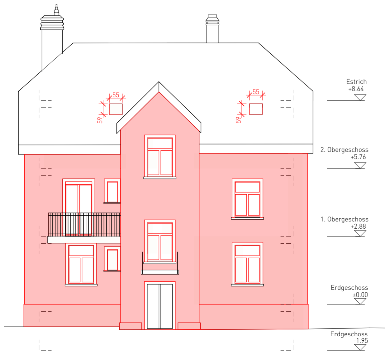
SÜDFASSADE MST. 1:100
