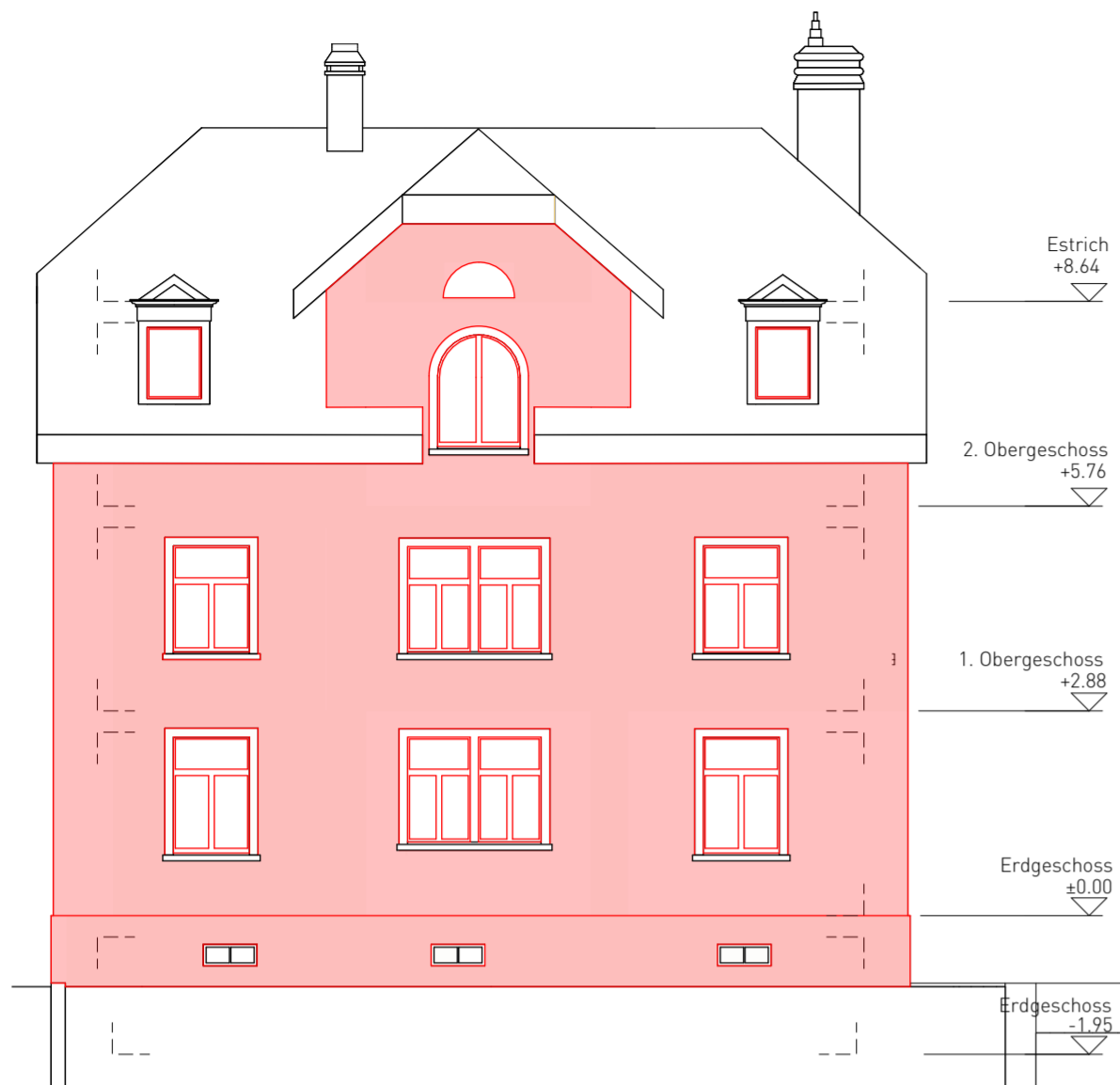
NORDFASSADE MST. 1:100
