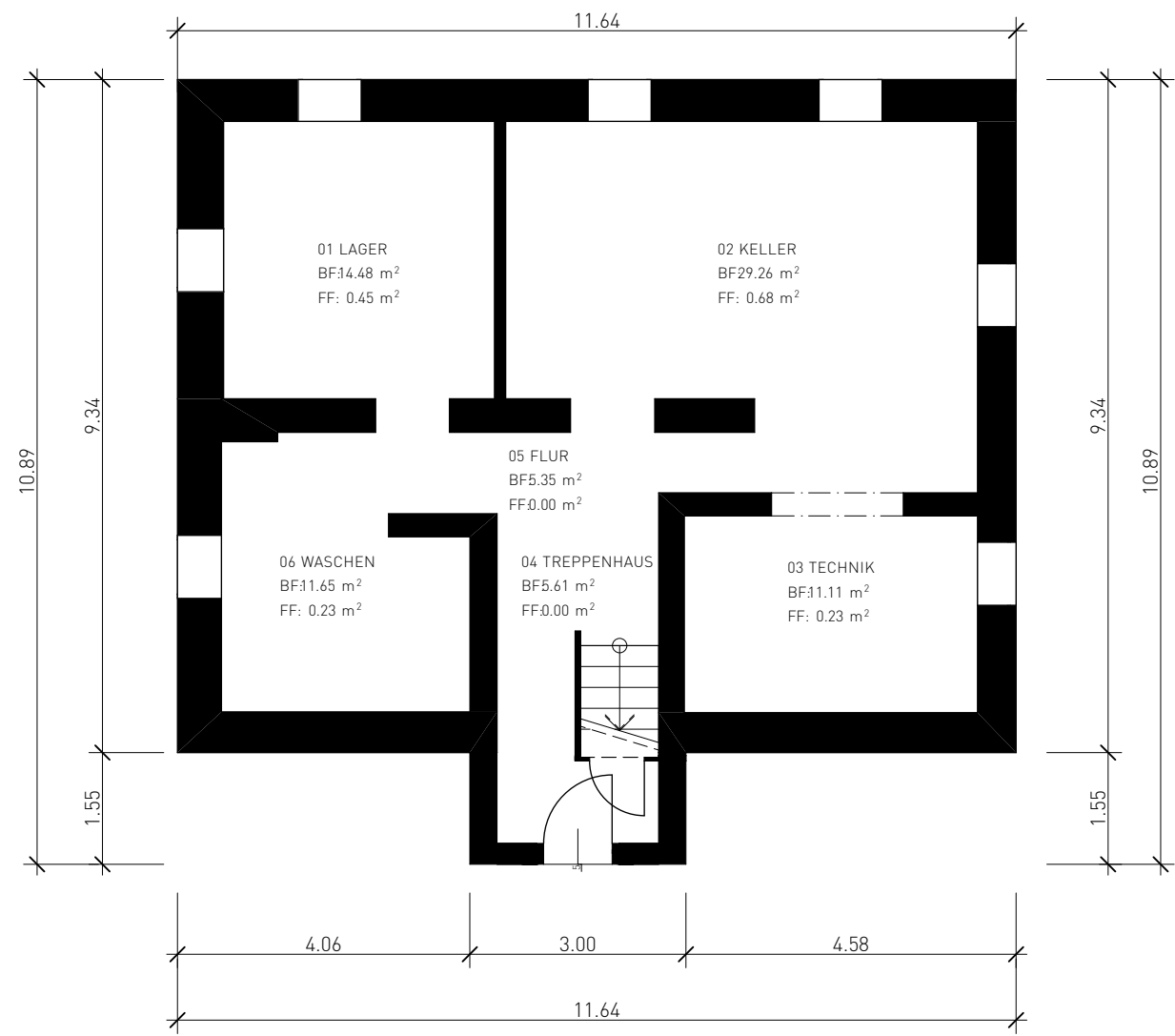
GRUNDRISS UG MST. 1:100
