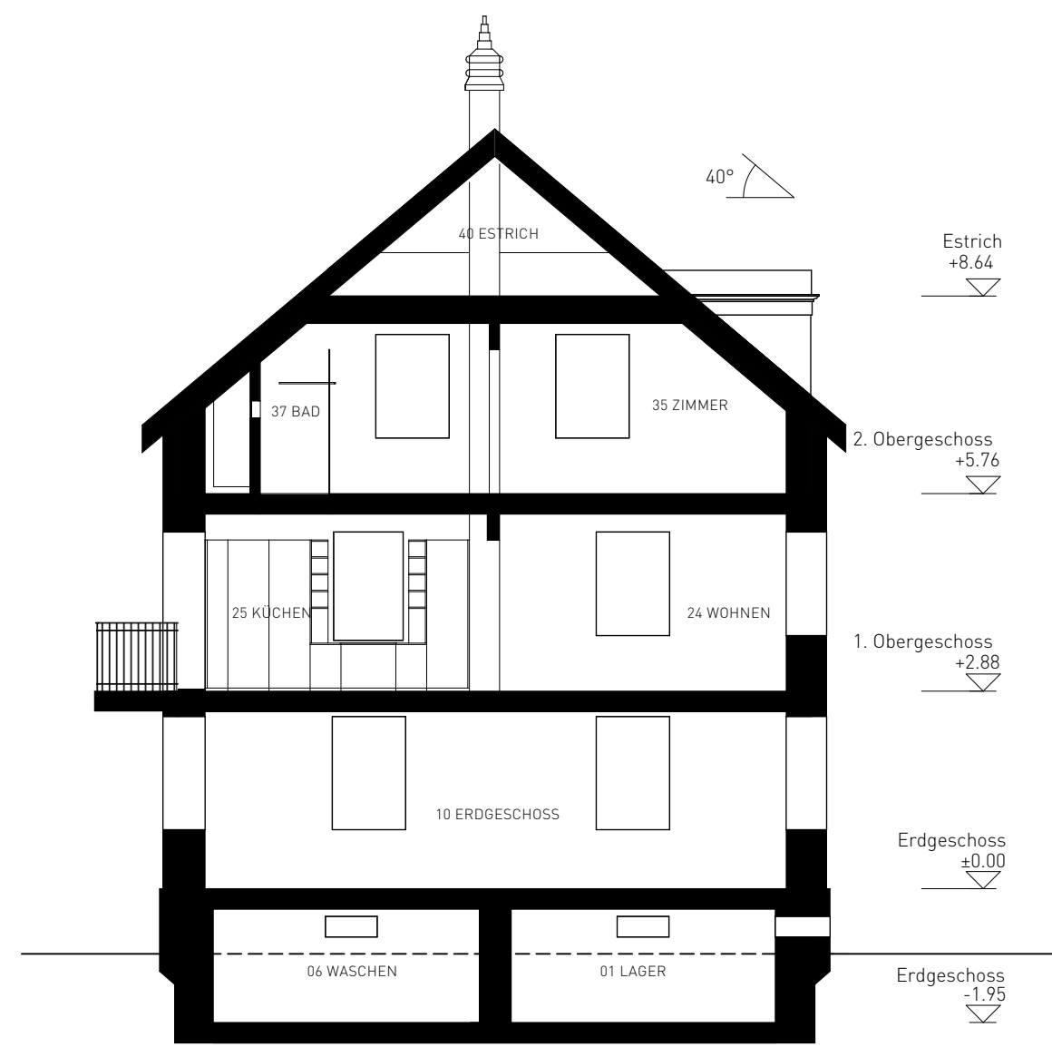
SCHNITT MST. 1:100
