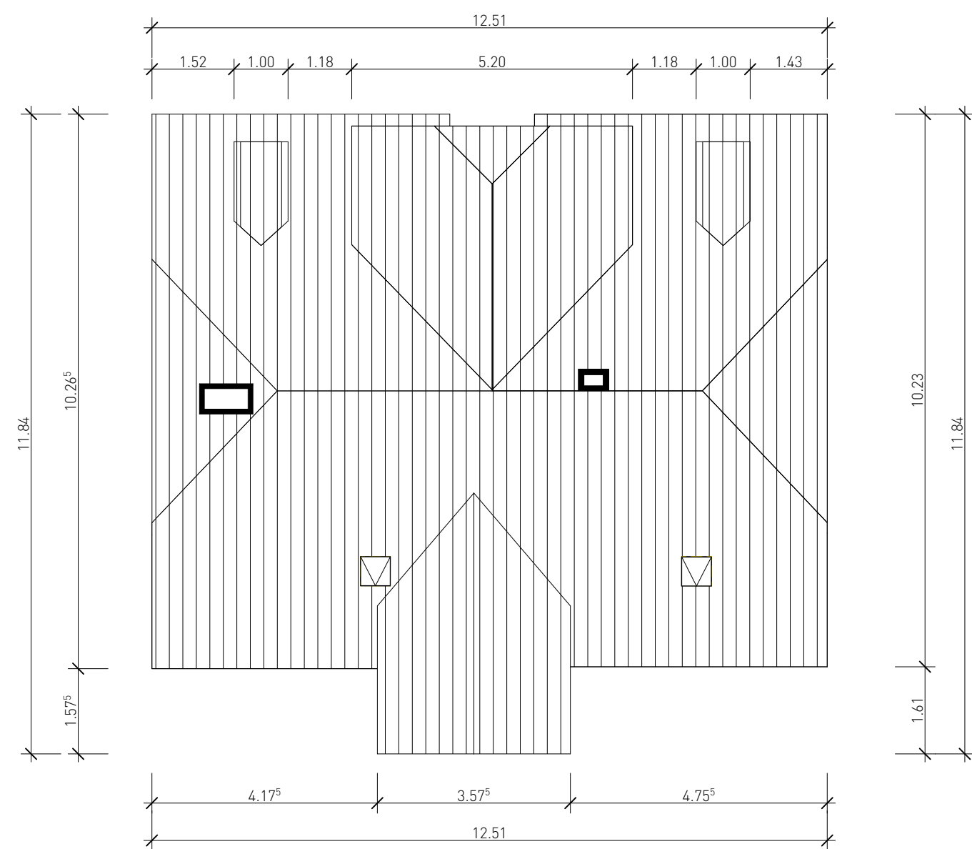
DACHAUFSICHT MST. 1:100
