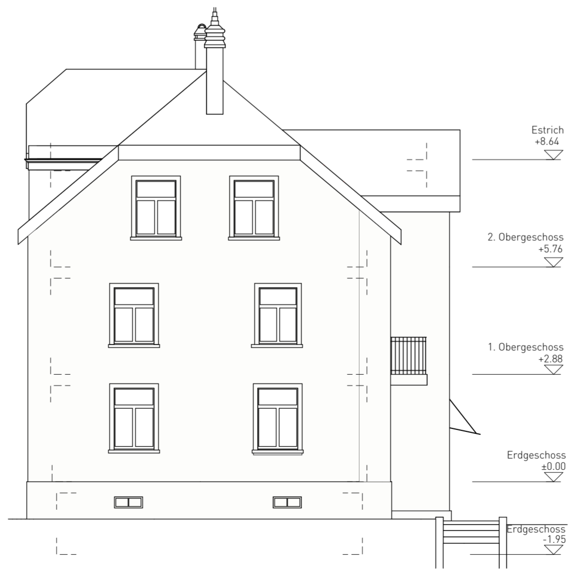
WESTFASSADE MST. 1:100
