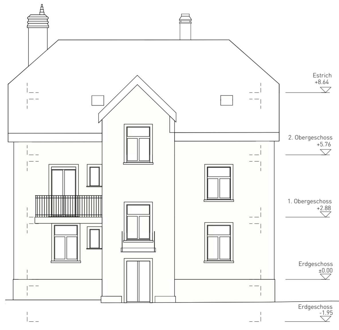
SÜDFASSADE MST. 1:100
