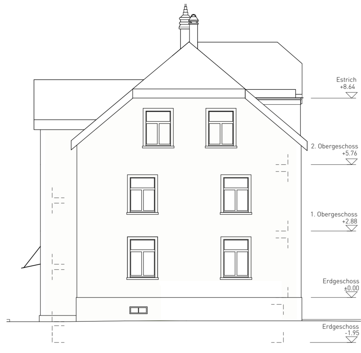
OSTFASSADE MST. 1:100
